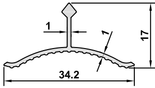
7221 AĞIRLIK / WEIGHT 0,149 kg/m
