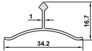
7222 AĞIRLIK / WEIGHT 0,141 kg/m
