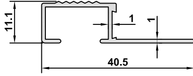
2203 AĞIRLIK / WEIGHT 0,192 kg/m
