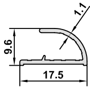
6485 AĞIRLIK / WEIGHT 0,100 kg/m
