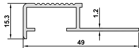
6121 AĞIRLIK / WEIGHT 0,303 kg/m
