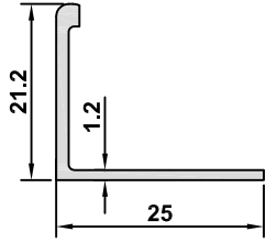
2258 AĞIRLIK / WEIGHT 0,171/m
