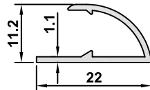
5125 AĞIRLIK / WEIGHT 0,130 kg/m
