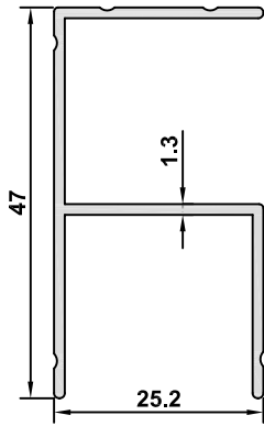
DK-58 AĞIRLIK / WEIGHT 0,404 kg/m
