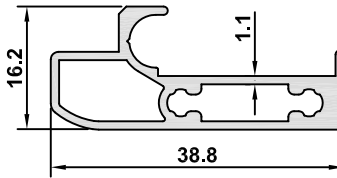
DK-23 AĞIRLIK / WEIGHT 0,410 kg/m
