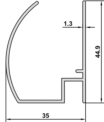
DK-14 AĞIRLIK / WEIGHT 0,455 kg/m
