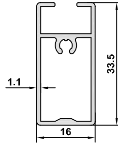
DK-04 AĞIRLIK / WEIGHT 0,347 kg/m
