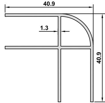
DK-16 AĞIRLIK / WEIGHT 0,518 kg/m
