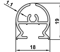
DK-17 AĞIRLIK / WEIGHT 0,239 kg/m
