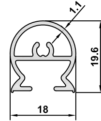
DK-02 AĞIRLIK / WEIGHT 0,255 kg/m
