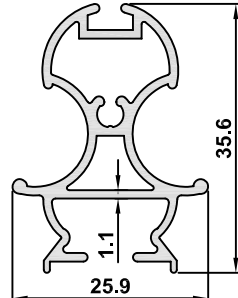
3204 AĞIRLIK / WEIGHT 0,455 kg/m
