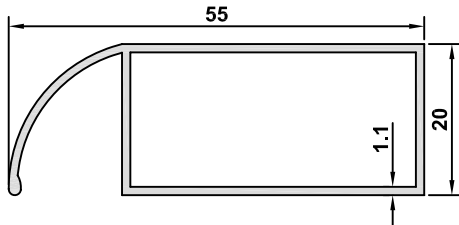
DK-22 AĞIRLIK / WEIGHT 0,426 kg/m
