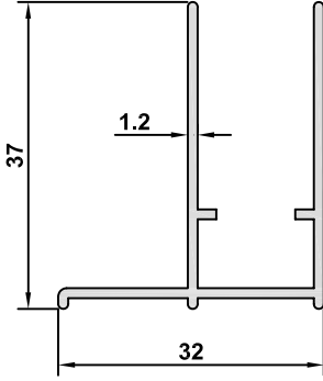
3202 AĞIRLIK / WEIGHT 0,352 kg/m
