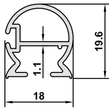
DK-01 AĞIRLIK / WEIGHT 0,241 kg/m
