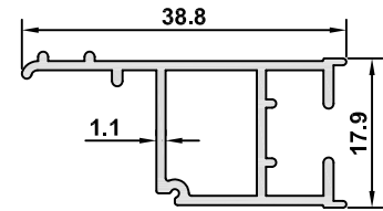
3216 AĞIRLIK / WEIGHT 0,328 kg/m
