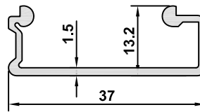
3201 AĞIRLIK / WEIGHT 0,282 kg/m
