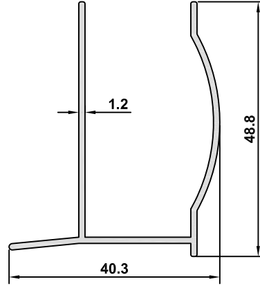
DK-18 AĞIRLIK / WEIGHT 0,423 kg/m
