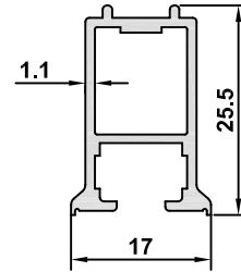
DK-10 AĞIRLIK / WEIGHT 0,277 kg/m
