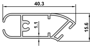
2554 AĞIRLIK / WEIGHT 0,363 kg/m
