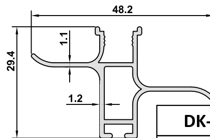
DK-60 AĞIRLIK / WEIGHT 0,404 kg/m
