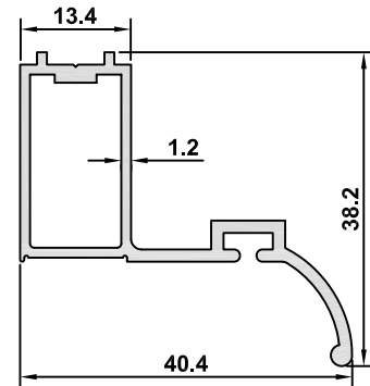
3200 AĞIRLIK / WEIGHT 0,442 kg/m
