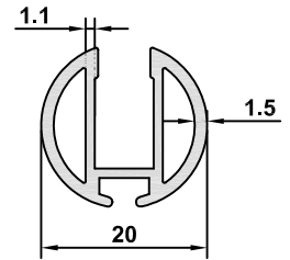
DK-21 AĞIRLIK / WEIGHT 0,315 kg/m
