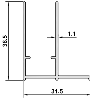
DK-09 AĞIRLIK / WEIGHT 0,317 kg/m
