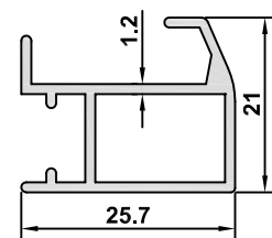
DK-53 AĞIRLIK / WEIGHT 0,315 kg/m
