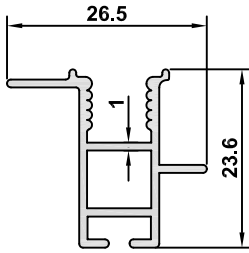
DK-64 AĞIRLIK / WEIGHT 0,268 kg/m
