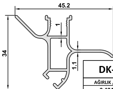
3215 AĞIRLIK / WEIGHT 0,141 kg/m
