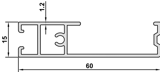
3217 AĞIRLIK / WEIGHT 0,488 kg/m
