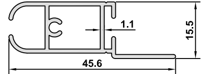
2553 AĞIRLIK / WEIGHT 0,350 kg/m
