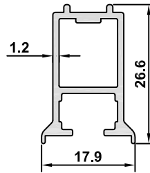
3206 AĞIRLIK / WEIGHT 0,295 kg/m
