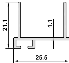
DK-56 AĞIRLIK / WEIGHT 0,208 kg/m
