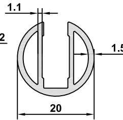
DK-20 AĞIRLIK / WEIGHT 0,317 kg/m
