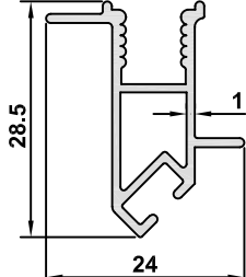
DK-65 AĞIRLIK / WEIGHT 0,276 kg/m
