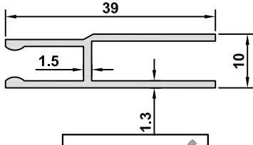
4670 AĞIRLIK / WEIGHT 0,312 kg/m
