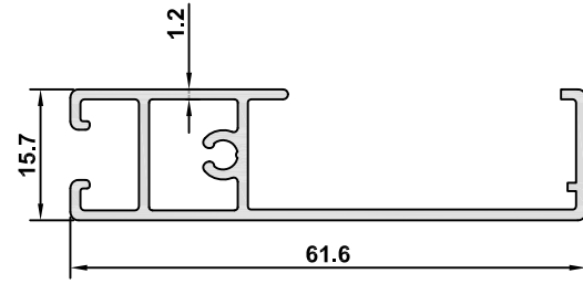
3211 AĞIRLIK / WEIGHT 0,496 kg/m
