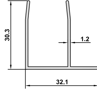
DK-15 AĞIRLIK / WEIGHT 0,282 kg/m
