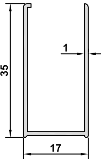
2555 AĞIRLIK / WEIGHT 0,230 kg/m
