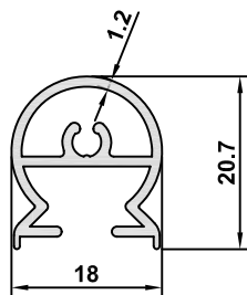
3209 AĞIRLIK / WEIGHT 0,279 kg/m
