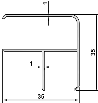
2557 AĞIRLIK / WEIGHT 0,323 kg/m
