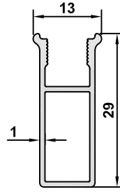
DK-54 AĞIRLIK / WEIGHT 0,222 kg/m
