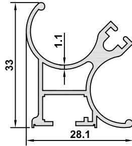
DK-05 AĞIRLIK / WEIGHT 0,436 kg/m
