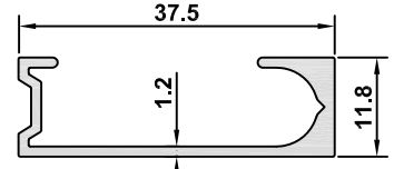
6464 AĞIRLIK / WEIGHT 0,280 kg/m
