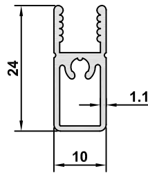
DK-50 AĞIRLIK / WEIGHT 0,239 kg/m
