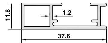
3213 AĞIRLIK / WEIGHT 0,331 kg/m
