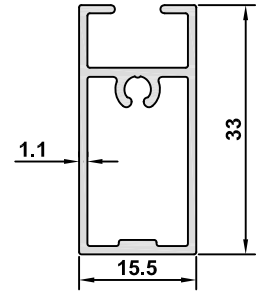
3205 AĞIRLIK / WEIGHT 0,342 kg/m
