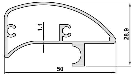
DK-13 AĞIRLIK / WEIGHT 0,575 kg/m
