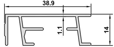
2558 AĞIRLIK / WEIGHT 0,306 kg/m
