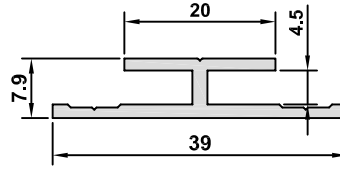
6869-18 AĞIRLIK / WEIGHT 0,284 kg/m
