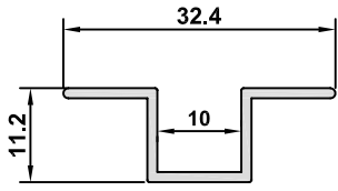
2651-12 AĞIRLIK / WEIGHT 0,171 kg/m
