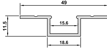
5061-15 AĞIRLIK / WEIGHT 0,285 kg/m
