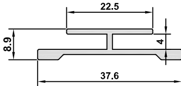
5204-15 AĞIRLIK / WEIGHT 0,344 kg/m
