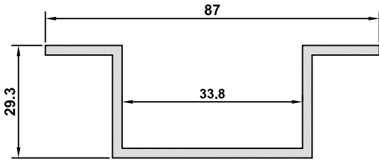
4627-25 AĞIRLIK / WEIGHT 0,955 kg/m
