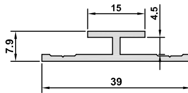
4993-1.6 AĞIRLIK / WEIGHT 0,266 kg/m
