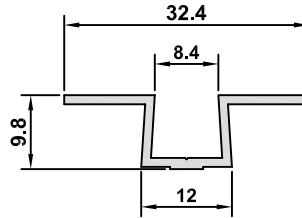
3078-12 AĞIRLIK / WEIGHT 0,168 kg/m
