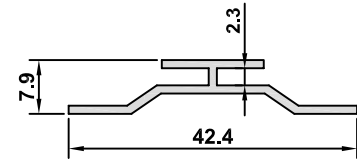
5259-12 AĞIRLIK / WEIGHT 0,205 kg/m
