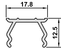
2198-15 AĞIRLIK / WEIGHT 0,140 kg/m
