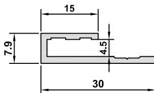
4995-1.6 AĞIRLIK / WEIGHT 0,217 kg/m
