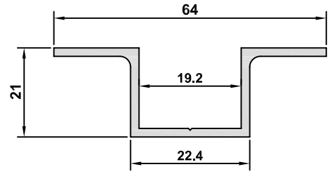
4481-20 AĞIRLIK / WEIGHT 0,561 kg/m
