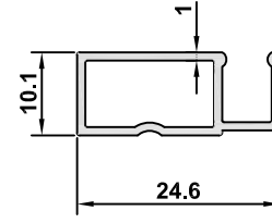
4260 AĞIRLIK / WEIGHT 0,187 kg/m
