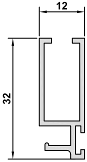
3012-12 AĞIRLIK / WEIGHT 0,379 kg/m
