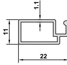
3013 AĞIRLIK / WEIGHT 0,193 kg/m
