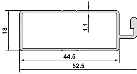
4658 AĞIRLIK / WEIGHT 0,434 kg/m
