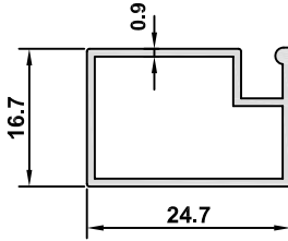
5967 AĞIRLIK / WEIGHT 0,222 kg/m
