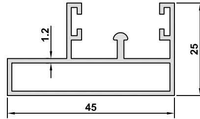
4205 AĞIRLIK / WEIGHT 0,542 kg/m
