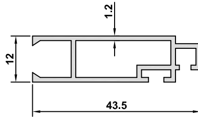
3012 AĞIRLIK / WEIGHT 0,401 kg/m
