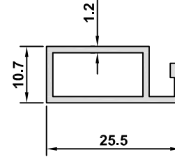
4449 AĞIRLIK / WEIGHT 0,228 kg/m
