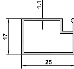
3060 AĞIRLIK / WEIGHT 0,257 kg/m
