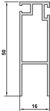
4204-12 AĞIRLIK / WEIGHT 0,450 kg/m
