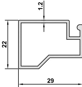
3107 AĞIRLIK / WEIGHT 0,331 kg/m
