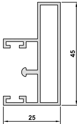
4205-12 AĞIRLIK / WEIGHT 0,512 kg/m
