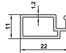
3013-1.2 AĞIRLIK / WEIGHT 0,220 kg/m
