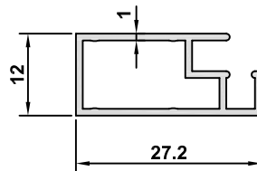
4669 AĞIRLIK / WEIGHT 0,220 kg/m
