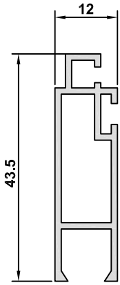
3012-12 AĞIRLIK / WEIGHT 0,379 kg/m
