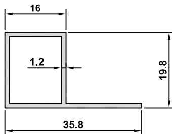
4657 AĞIRLIK / WEIGHT 0,282 kg/m
