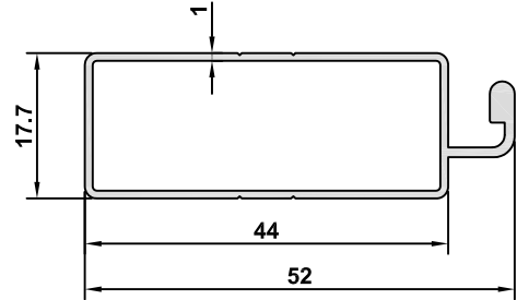
4751 AĞIRLIK / WEIGHT 0,374 kg/m
