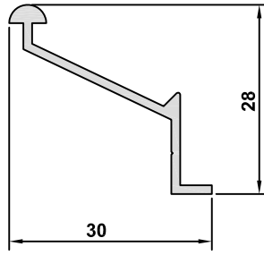
3011-12 AĞIRLIK / WEIGHT 0,198 kg/m
