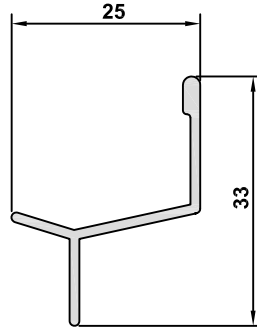
4303-12 AĞIRLIK / WEIGHT 0,205 kg/m
