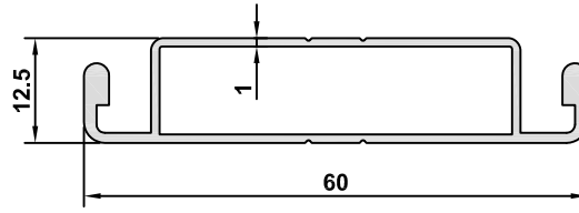
4656 AĞIRLIK / WEIGHT 0,442 kg/m
