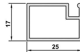
3060-1.2 AĞIRLIK / WEIGHT 0,290 kg/m
