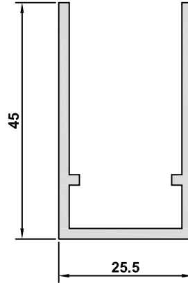
4461 AĞIRLIK / WEIGHT 0,625 kg/m
