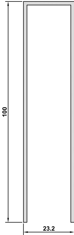
4733 AĞIRLIK / WEIGHT 0,950 kg/m
