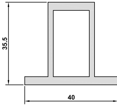
4635 AĞIRLIK / WEIGHT 0,920 kg/m
