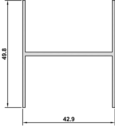
3092-12 AĞIRLIK / WEIGHT 0,520 kg/m
