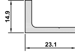
4793 AĞIRLIK / WEIGHT 0,257 kg/m
