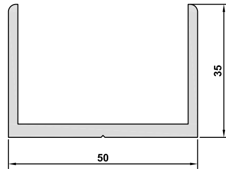
4149-00 AĞIRLIK / WEIGHT 0,894 kg/m
