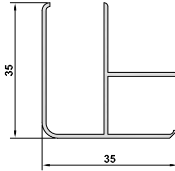
2557-00 AĞIRLIK / WEIGHT 0,320 kg/m
