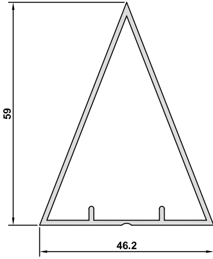
4200 AĞIRLIK / WEIGHT 0,607 kg/m
