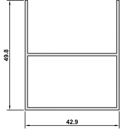
3091-12 AĞIRLIK / WEIGHT 0,610 kg/m
