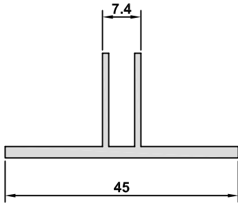
4795 AĞIRLIK / WEIGHT 0,384 kg/m
