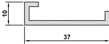
4739-2.0 AĞIRLIK / WEIGHT 0,287 kg/m
