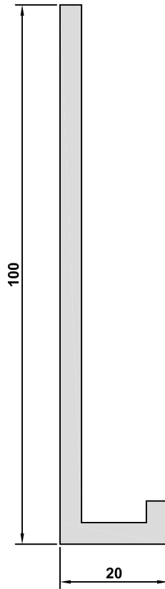
3085 AĞIRLIK / WEIGHT 1,301 kg/m
