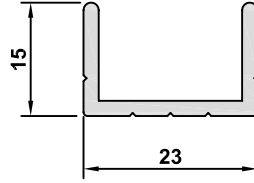
4445 AĞIRLIK / WEIGHT 0,260 kg/m
