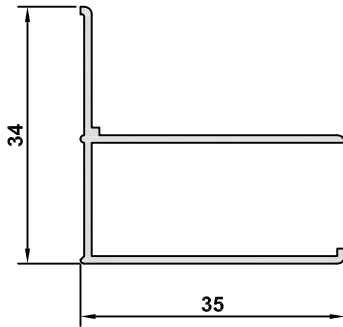
2556-12 AĞIRLIK / WEIGHT 0,282 kg/m
