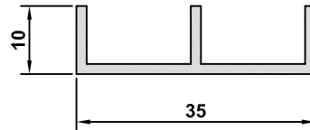
5058-1.5 AĞIRLIK / WEIGHT 0,805 kg/m
