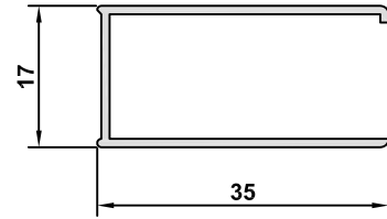
2555-12 AĞIRLIK / WEIGHT 0,230 kg/m
