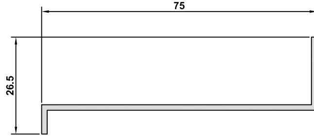
5922 AĞIRLIK / WEIGHT 0,407 kg/m
