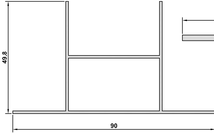
4874-12 AĞIRLIK / WEIGHT 0,745 kg/m
