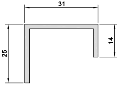
5230-2.0 AĞIRLIK / WEIGHT 0358 kg/m
