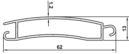
3614 AĞIRLIK / WEIGHT 0,455 kg/m
