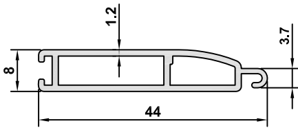
3612 AĞIRLIK / WEIGHT 0,331 kg/m
