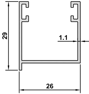
2018 AĞIRLIK / WEIGHT 0,287kg/m
