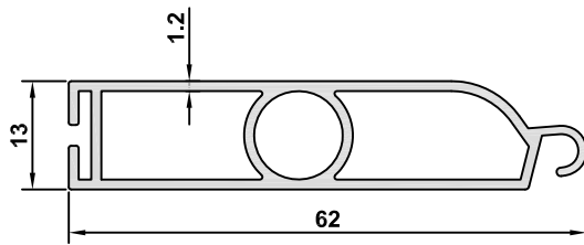
3608 AĞIRLIK / WEIGHT 0,566 kg/m
