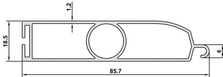
3603 AĞIRLIK / WEIGHT 0,832 kg/m
