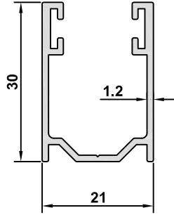
3613 AĞIRLIK / WEIGHT 0,342 kg/m
