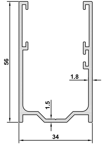
3607 AĞIRLIK / WEIGHT 0,745 kg/m
