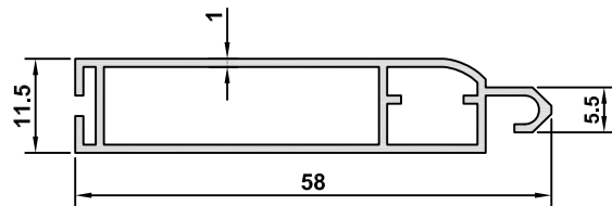
4240 AĞIRLIK / WEIGHT 0,409 kg/m
