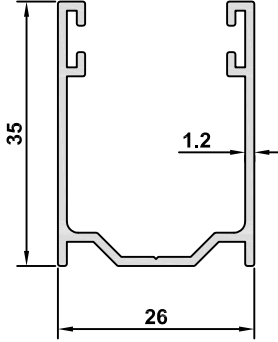
3609 AĞIRLIK / WEIGHT 0,371 kg/m
