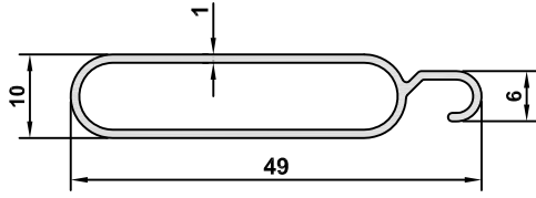
2202 AĞIRLIK / WEIGHT 0,282 kg/m
