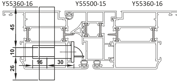
İÇE AÇILIR KAPI / INWARD OPENING DOOR
