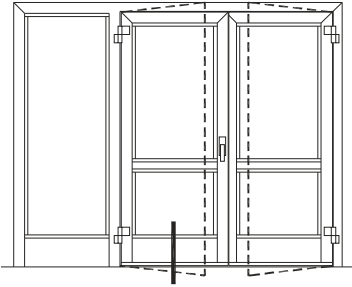
İÇE AÇILIR BİNİLİ KAPI
