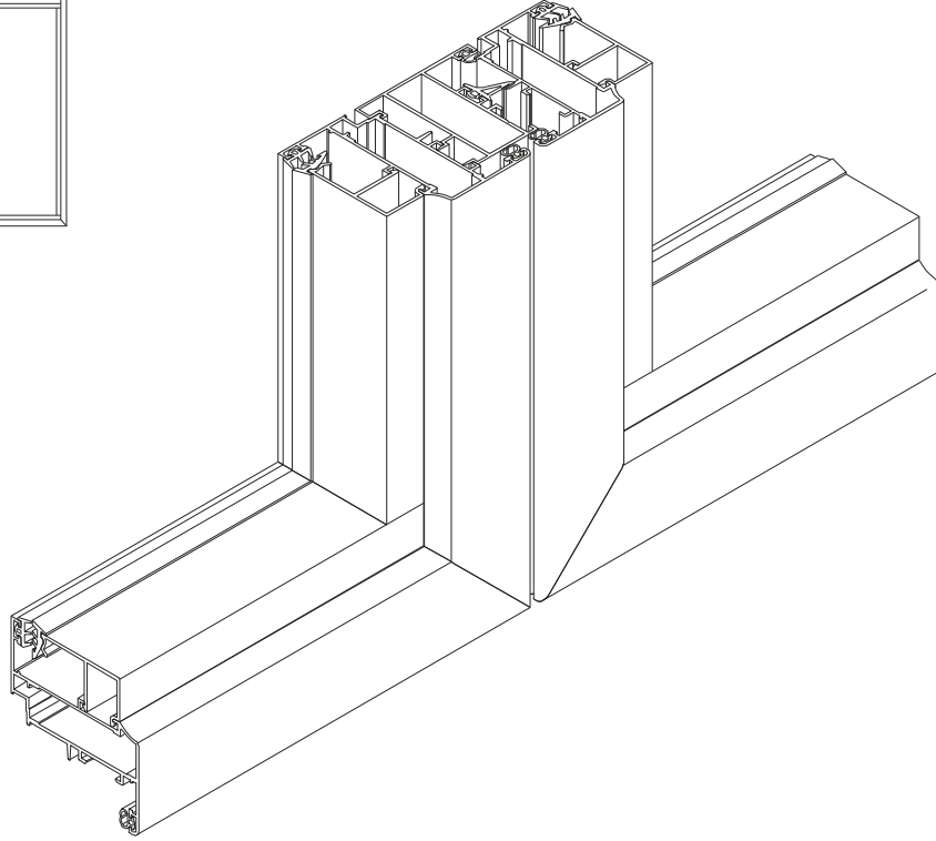
İÇE AÇILIR PENCERE INWARD OPENING WINDOW
