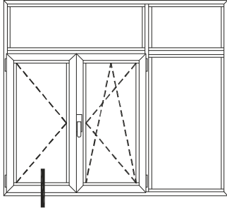
İÇE AÇILIR PENCERE INWARD OPENING WINDOW
