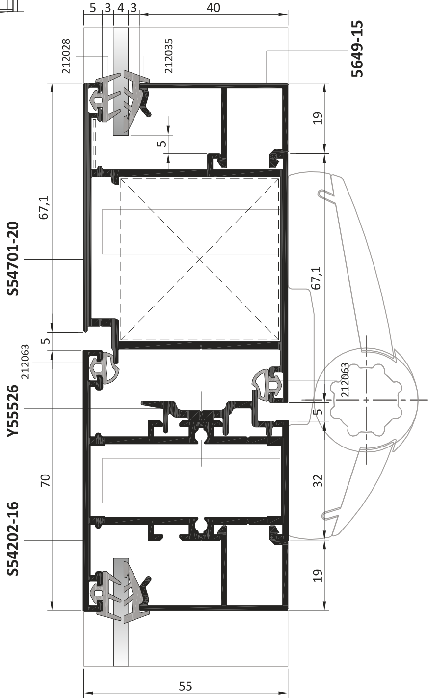
İÇE AÇILIR HEMYÜZ KAPI INWARD OPENING FLUSH DOOR
