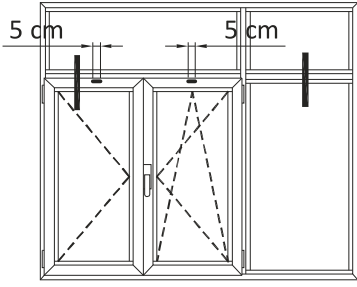
İÇE AÇILIR PENCERE INWARD OPENING WINDOW
