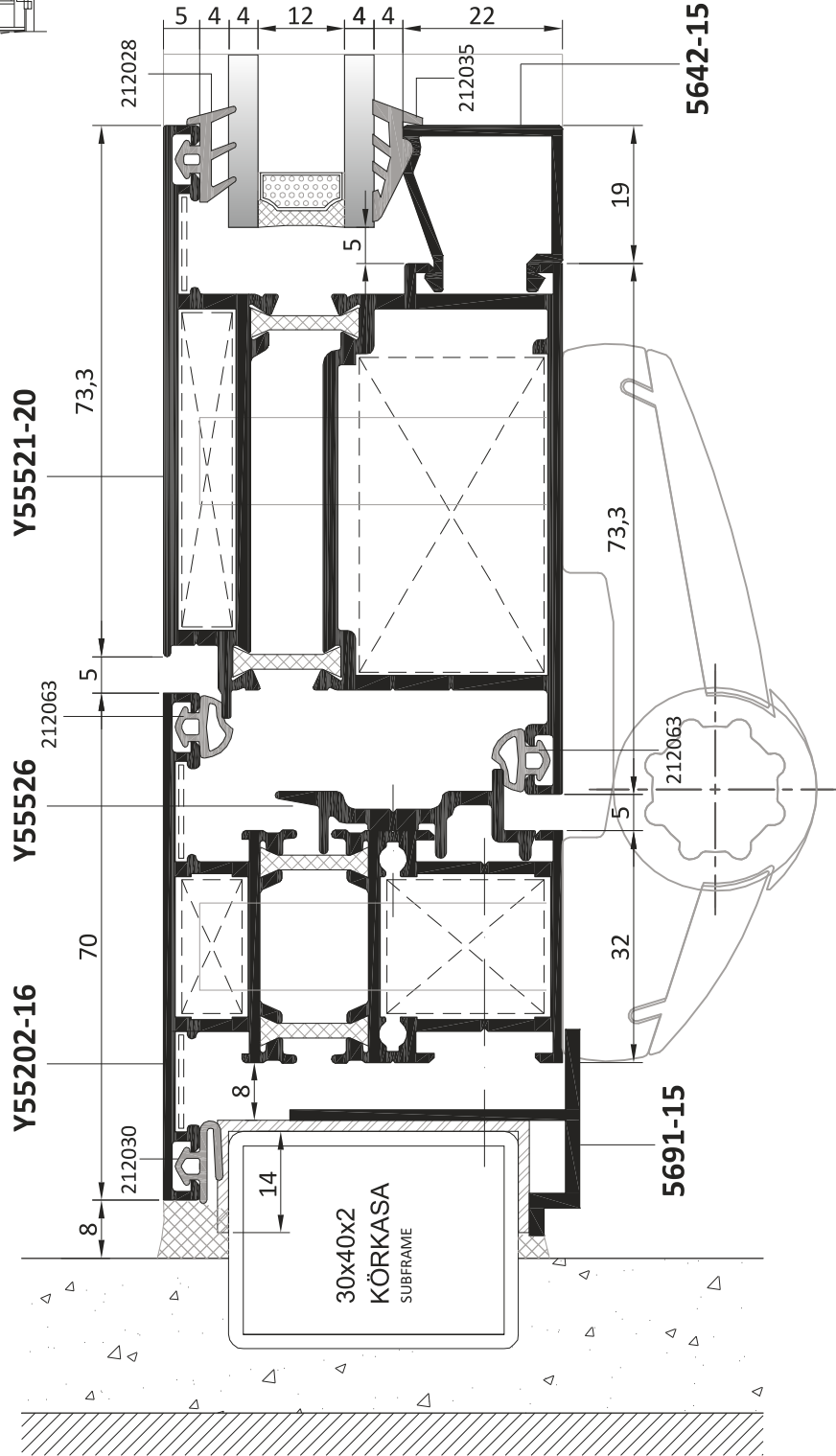
İÇE AÇILIR HEMYÜZ KAPI INWARD OPENING FLUSH DOOR
