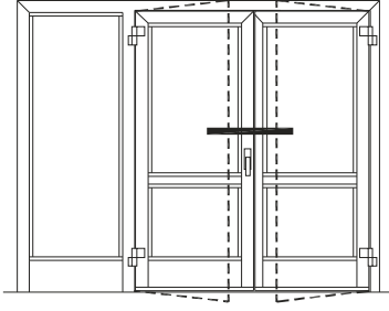
İÇE AÇILIR HEMYÜZ KAPI INWARD OPENING FLUSH DOOR
