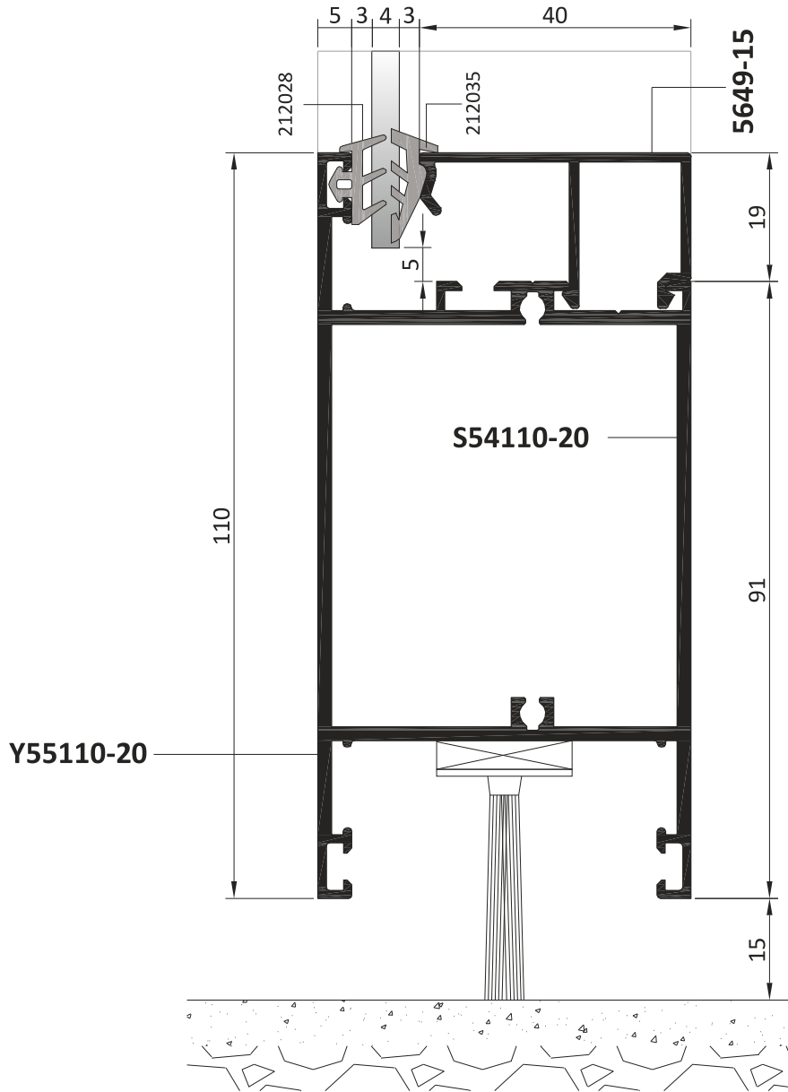
İÇE AÇILIR HEMYÜZ KAPI INWARD OPENING FLUSH DOOR
