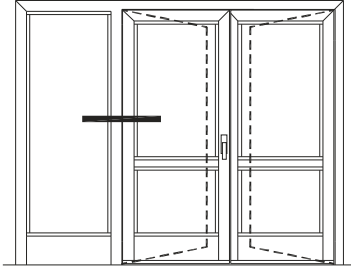
DIŞA AÇILIR HEMYÜZ KAPI OUTWARD OPENING FLUSH DOOR
