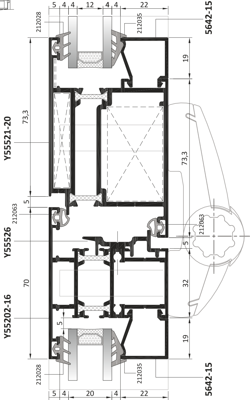
İÇE AÇILIR HEMYÜZ KAPI INWARD OPENING FLUSH DOOR
