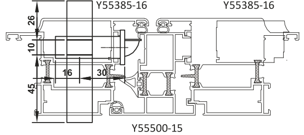
DIŞA AÇILIR KAPI / OUTWARD OPENING DOOR
