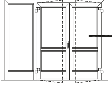
İÇE AÇILIR HEMYÜZ KAPI INWARD OPENING FLUSH DOOR
