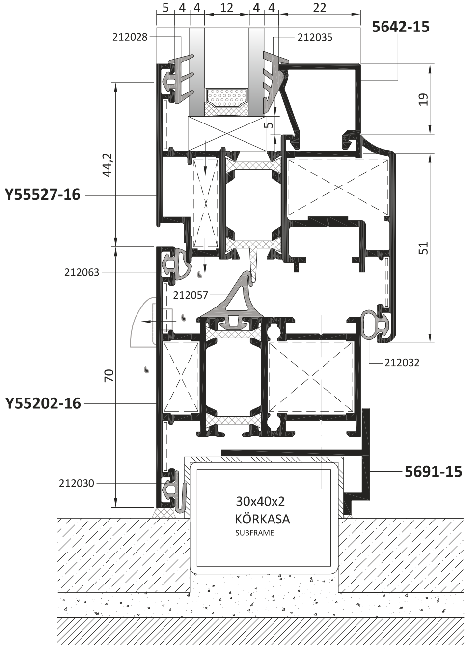
İÇE AÇILIR PENCERE INWARD OPENING WINDOW
