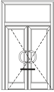
ÇARPMA KAPI SWING DOOR
