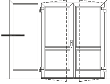
İÇE AÇILIR HEMYÜZ KAPI INWARD OPENING FLUSH DOOR
