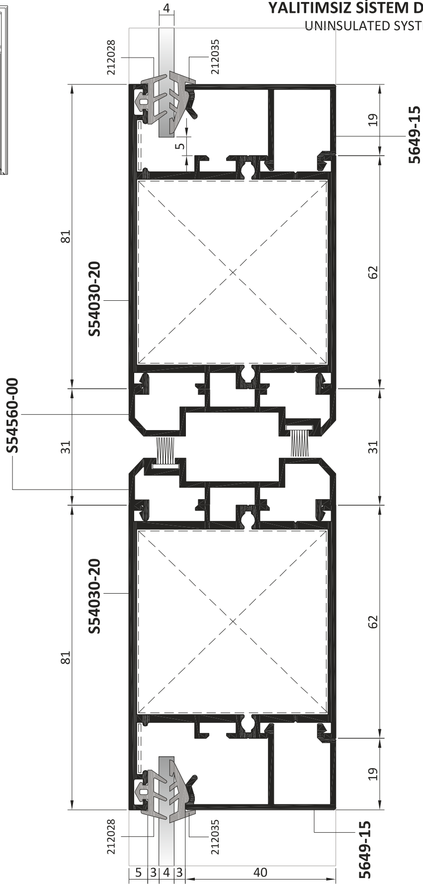
ÇARPMA KAPI SWING DOOR
