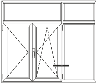
İÇE AÇILIR PENCERE INWARD OPENING WINDOW
