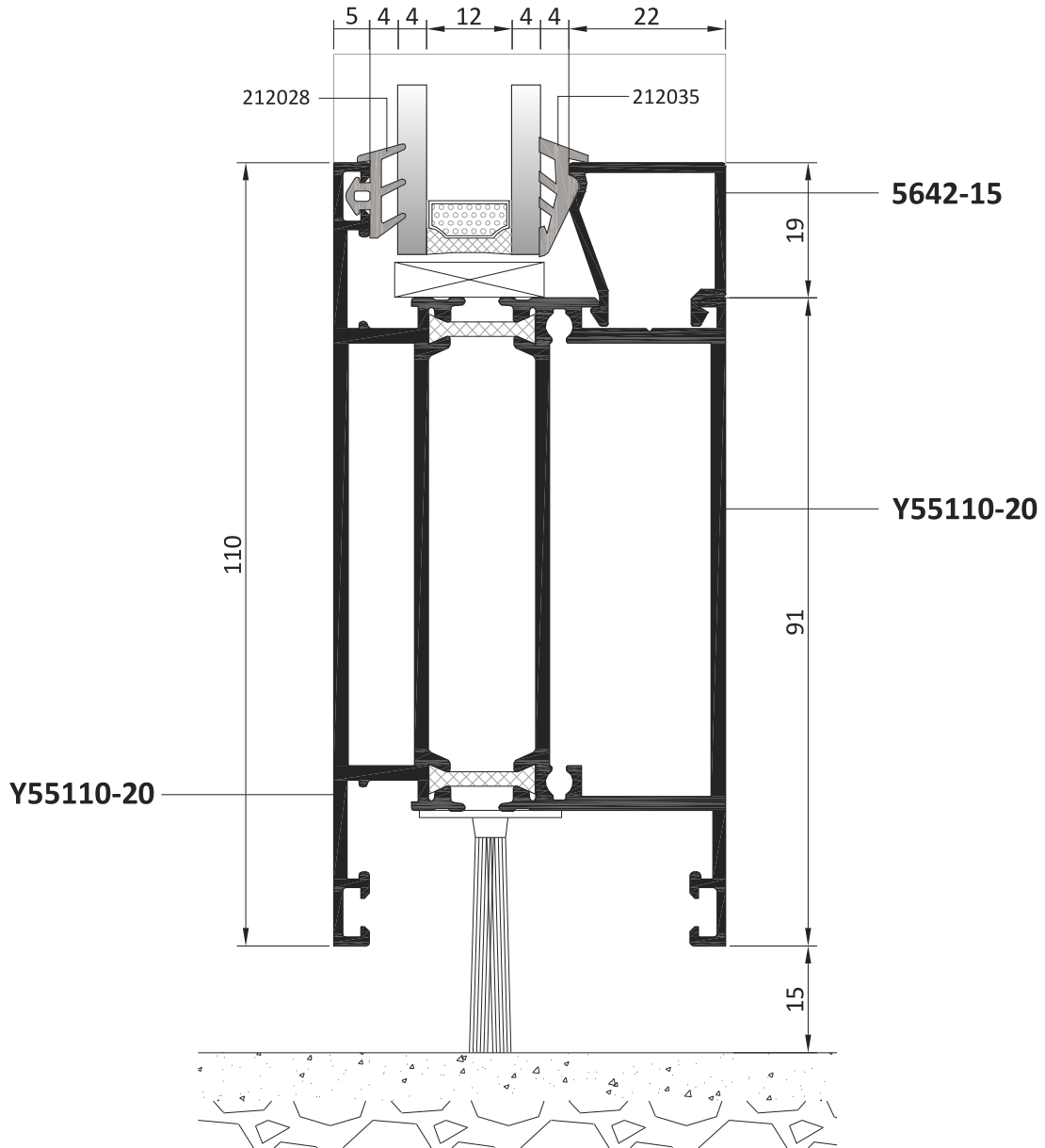
İÇE AÇILIR HEMYÜZ KAPI INWARD OPENING FLUSH DOOR
