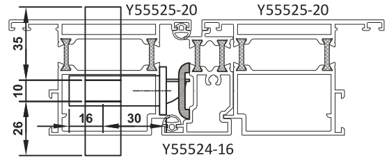
DIŞA AÇILIR KAPI / OUTWARD OPENING DOOR
