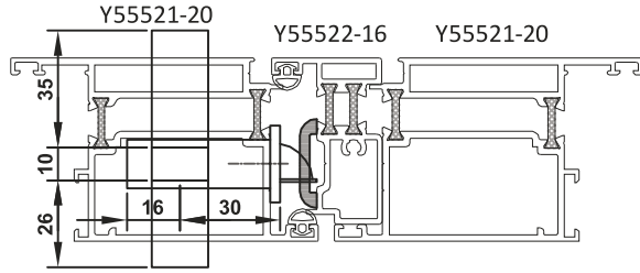
İÇE AÇILIR KAPI / INWARD OPENING DOOR
