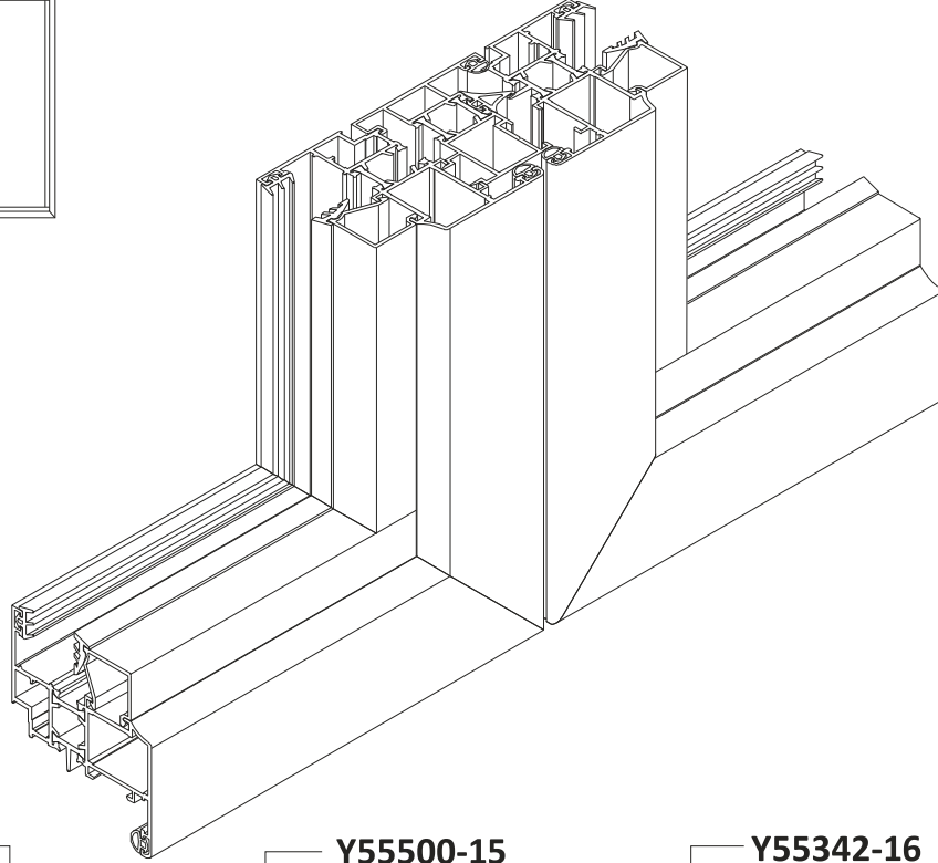
İÇE AÇILIR PENCERE INWARD OPENING WINDOW
