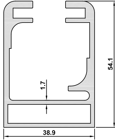
6386 AĞIRLIK / WEIGHT 1,412 kg/m
