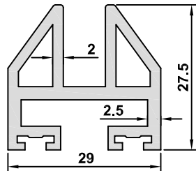
4767 AĞIRLIK / WEIGHT 0,772 kg/m
