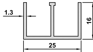
2022 AĞIRLIK / WEIGHT 0,249 kg/m
