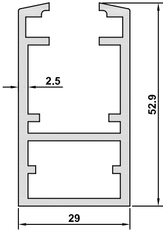
4750 AĞIRLIK / WEIGHT 1,133 kg/m
