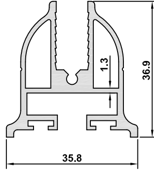
6385 AĞIRLIK / WEIGHT 0,795 kg/m
