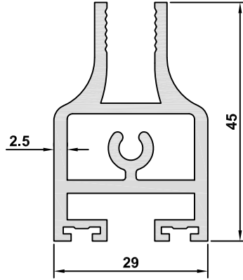
4749 AĞIRLIK / WEIGHT 1,103 kg/m
