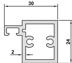
4778 AĞIRLIK / WEIGHT 0,591 kg/m
