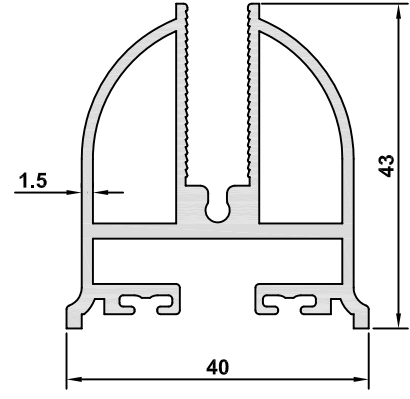
6966 AĞIRLIK / WEIGHT 1,024 kg/m
