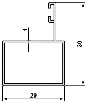
6876 AĞIRLIK / WEIGHT 0,330 kg/m
