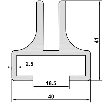
4896 AĞIRLIK / WEIGHT 1,168 kg/m
