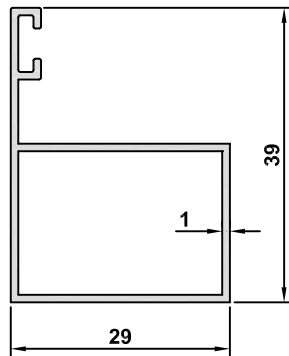
5528 AĞIRLIK / WEIGHT 0,336 kg/m
