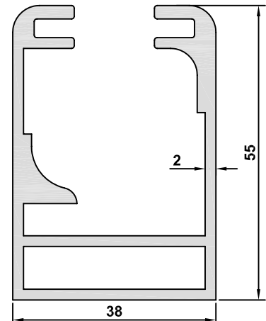
4844 AĞIRLIK / WEIGHT 1,417 kg/m
