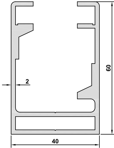
6967 AĞIRLIK / WEIGHT 1,458 kg/m
