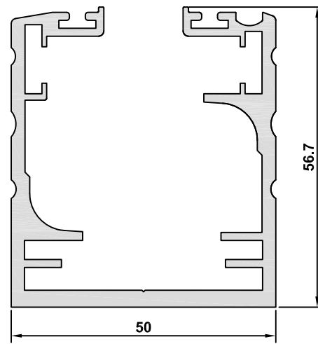
6932 AĞIRLIK / WEIGHT 1,674 kg/m
