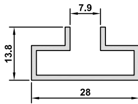
4684 AĞIRLIK / WEIGHT 0,250 kg/m
