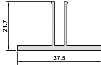
5043 AĞIRLIK / WEIGHT 0,352 kg/m
