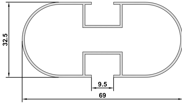
2072 AĞIRLIK / WEIGHT 0,604 kg/m
