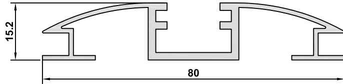
5173 AĞIRLIK / WEIGHT 0,691 kg/m
