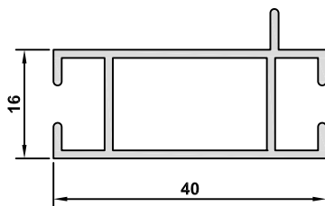
4346 AĞIRLIK / WEIGHT 0,420 kg/m
