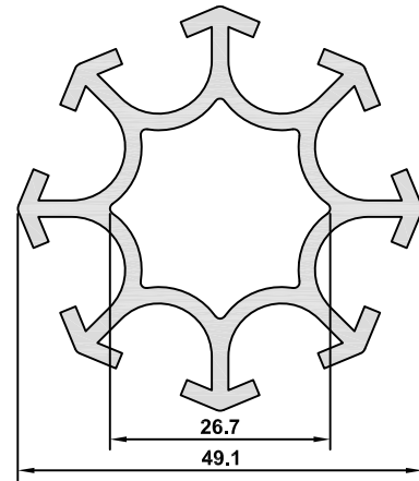
6637 AĞIRLIK / WEIGHT 1,250 kg/m
