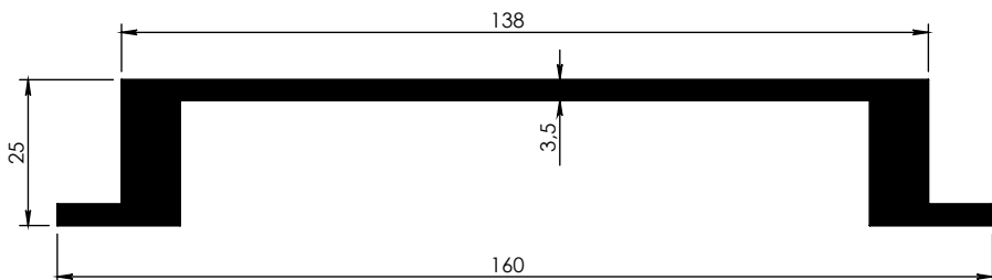
4488 - 2,697 kg/m
