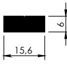
4801 - 0,255 kg/m
