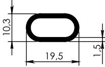
4806 - 0,190 kg/m
