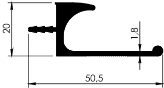
6205 - 0,525 kg/m
