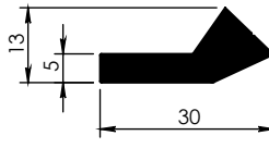
6204 - 0,488 kg/m
