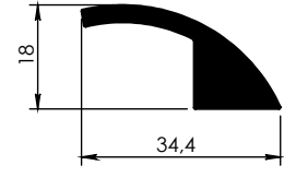
5148 - 0,553 kg/m
