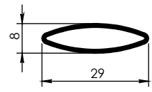
5232 - 0,163 kg/m
