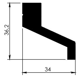
4487 - 0,979 kg/m
