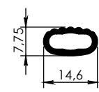
4807 - 0,122 kg/m
