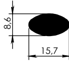
4802 - 0,280 kg/m
