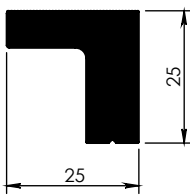
4884 - 0,955 kg/m
