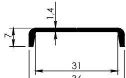
5973 - 0,190 kg/m
