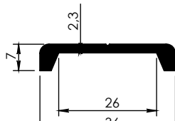
4110 - 0,320 kg/m
