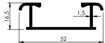
5070 - 0,412 kg/m
