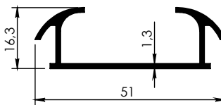
5069 - 0,353 kg/m
