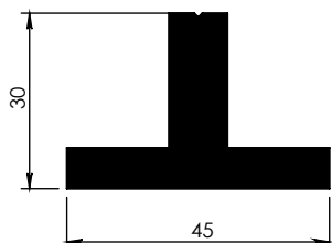
4485 - 1,480 kg/m
