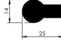
5035 - 0,664 kg/m
