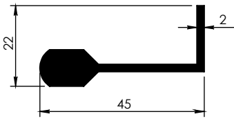
5089 - 0,613 kg/m
