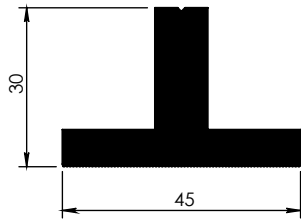
4486 - 1,460 kg/m
