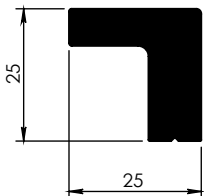
4883 - 0,962 kg/m
