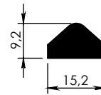
4803 - 0,280 kg/m
