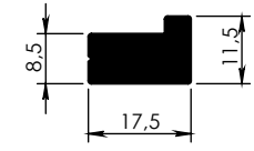
5402 - 0,439 kg/m
