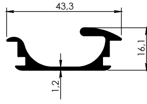
6240 - 0,412 kg/m
