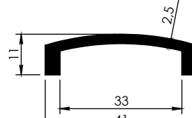
4116 - 0,412 kg/m
